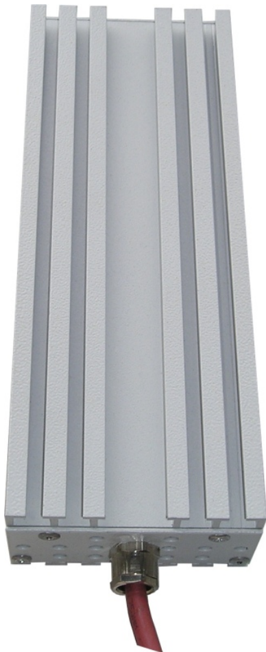
TypS-SerieSandwich-Widerstand.jpg
