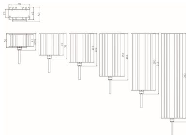
Typ-S---Serie-Sandwich-Zeichnung1.jpg
