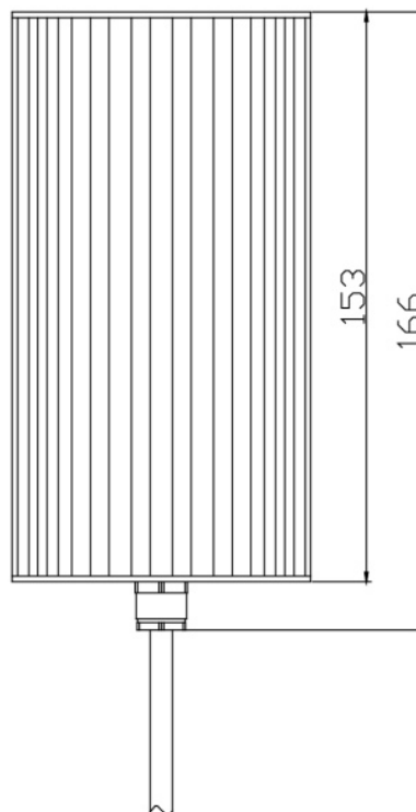
Typ2-LM-StandardWiderstand-Zeichnung.jpg
