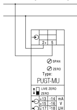
DC-Spannungsmessung DC-voltage measuring
