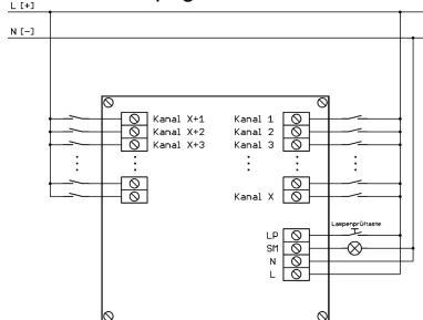
LM(B)T144-Anschluss.png
