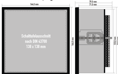
LM144_Gehaeuseseite_Befestigung.png
